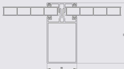
Coupe de la poutre
