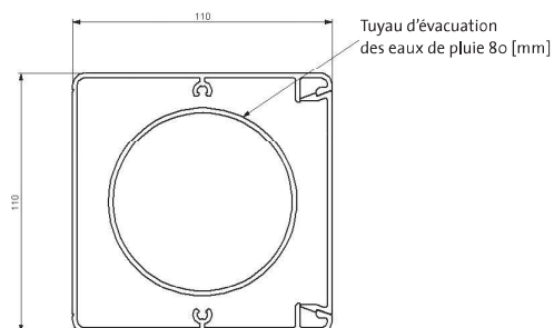
Coupe vue d'en haut d'un montant standard
