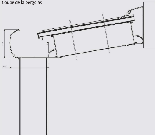
Coupe de la pergolas
